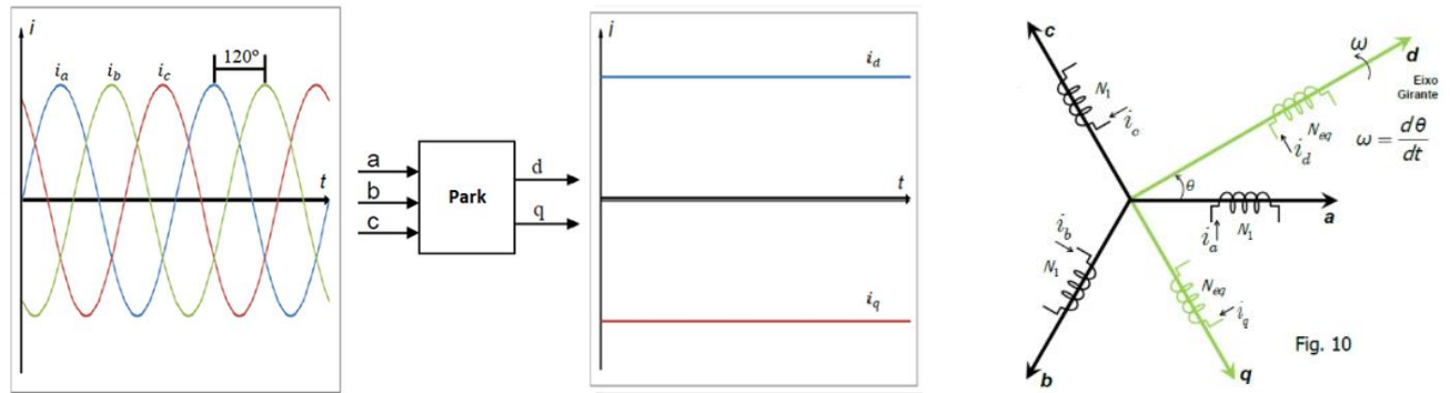
Figura 6: (izq.) Representación de la transformación de Park corrientes de fase, y su nueva representación en i_d e i_q . (der) Representación de los ejes longitudinal d, transversal q y perpendicular a ambos 0.
