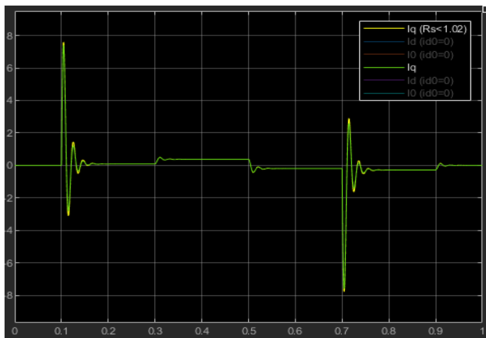
Figura 32: Comparación de corrientes para modelos NL(amarillo) y LTI (verde)
